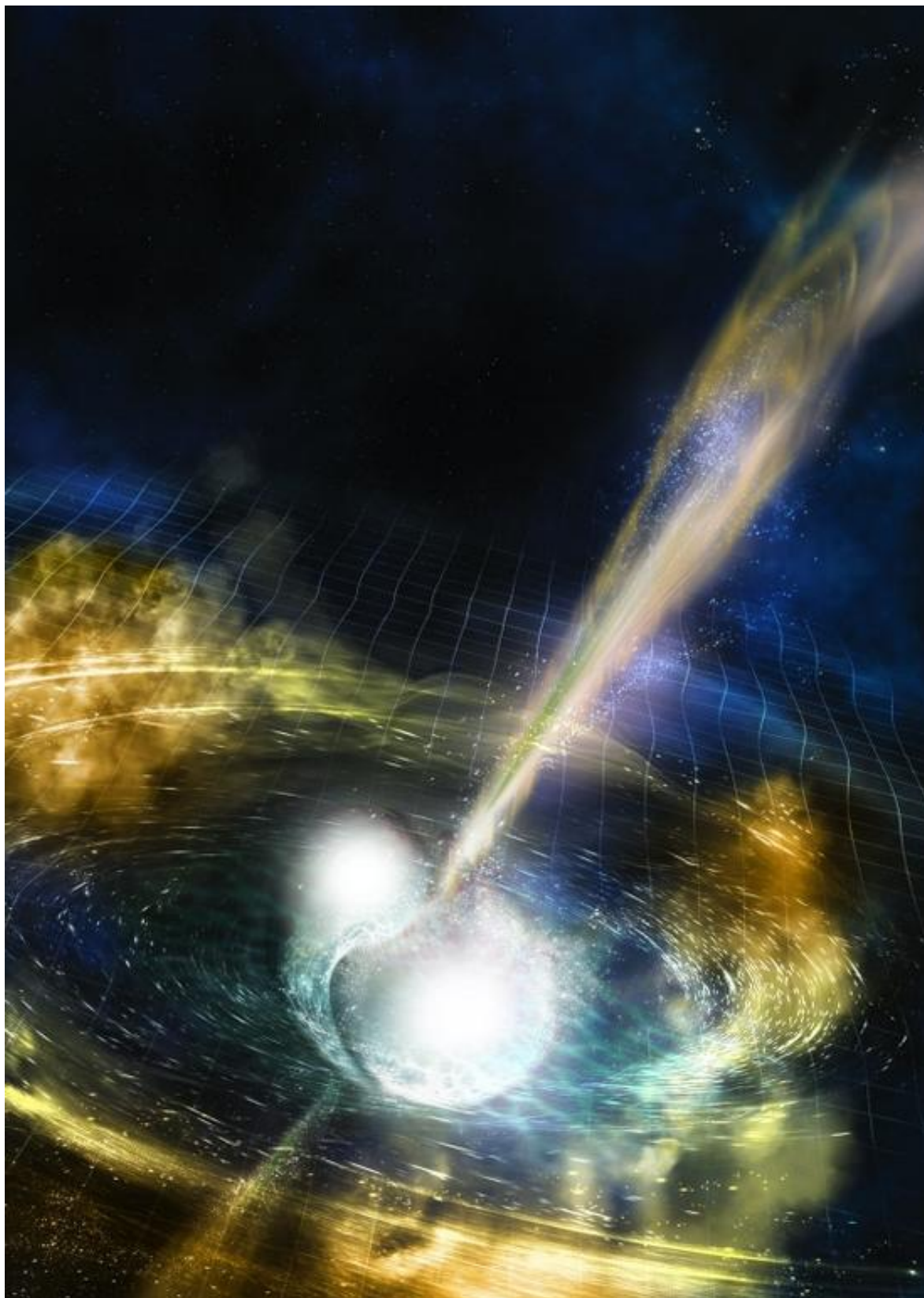
这张由美国国家科学基金会、美国“激光干涉引力波天文台”、索诺玛州立大学和A. Simonet提供的效果图显示的是两个合并中的中子星。新华社 图
